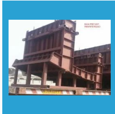
Parapete precast mould.
